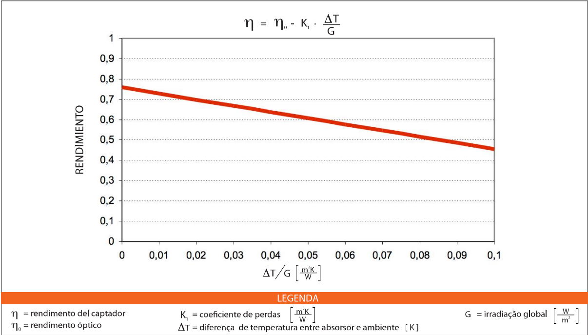
CURVA DE RENDIMENTO DO COLECTOR PLANO HORIZONTAL SELECTIVO OPS-H210 *
