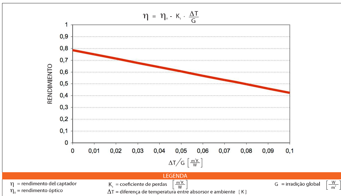
CURVA DE RENDIMENTO DO COLECTOR PLANO VERTICAL SELECTIVO OPS-V210 *
